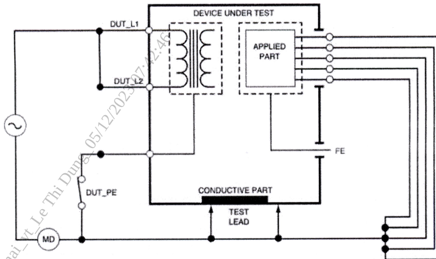
Hình 7. Sơ đồ nguyên lý của phép đo dòng điện rò thiết bị bằng phương pháp thay thế
